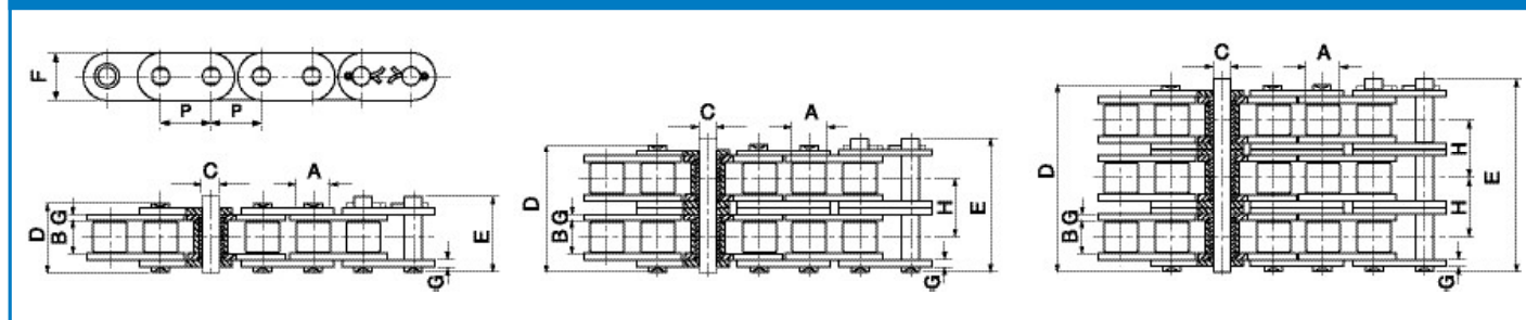
ANSI Válečkové řetězy s rovnými deskami
