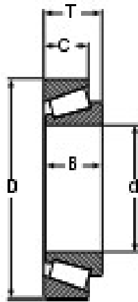
Metrická kuželíková ložiska
